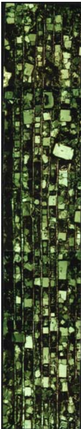
Серебряная лента с искусственным (полосчатым) рельефом поверхности, двуслоно-текстурирующим кристаллы ВТСП фазы YBa_2Cu_3O_x .
