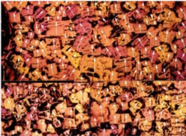
Структурно-чувствительные свойства ВТСП.
