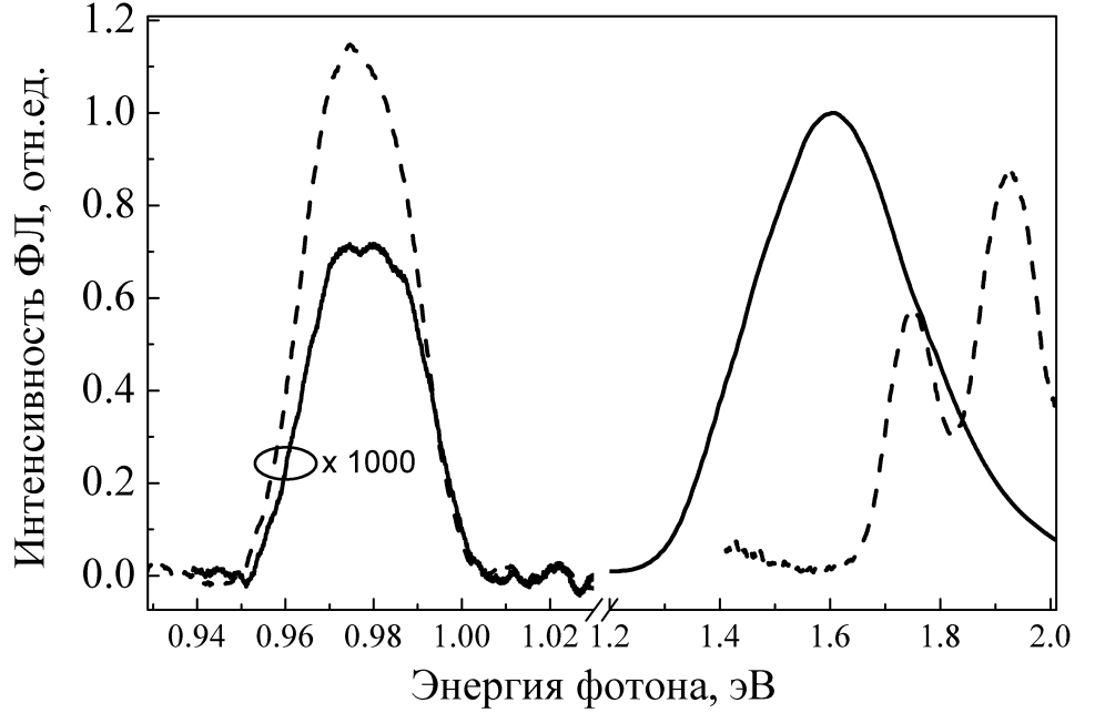
Рис. 4. Справа от разрыва оси: спектры фотолуминесценции порошков кремниевых нанокристаллов (сплошные кривые) и мезопорфирин-IX в тетрагидрометане (пунктир) в отсутствие молекул кислорода, слева от разрыва — спектры люминесценции сенсibilизированного ими синглетного кислорода в присутствии молекул кислорода.
