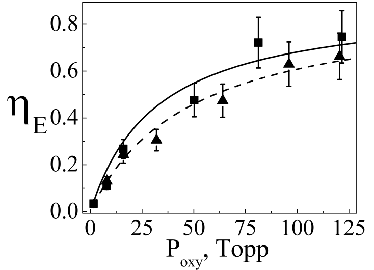
Рис. 5. Зависимость эффективности переноса энергии, \eta_E , в порошках (квадраты) и водных суспензиях (треугольники) кремниевых нанокристаллов от парциального давления кислорода P_{ox} и её аппроксимация в рамках модели мономолекулярной адсорбции Лэнгмюра (сплошная и пунктирная линии).
