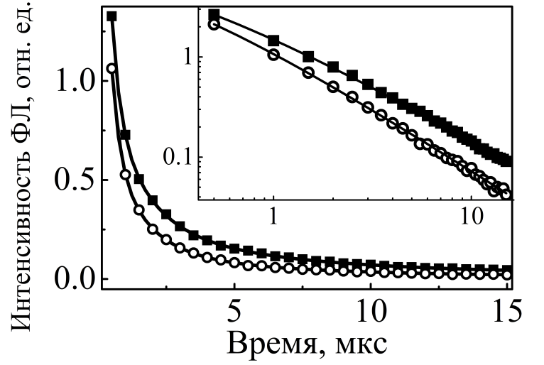
Рис. 7. Временные зависимости интенсивности люминесценции ^1O_2 , фотосенсибилизированного кремниевыми нанокристаллами в D_2O , без тушителя (квадраты) и после добавления 0.1 моль/л NaN_3 (окружности). На вставке показаны те же кривые в двойном логарифмическом масштабе. Сплошные линии — результат аппроксимации функцией (5).
