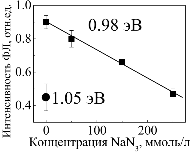
Рис. 6. Зависимость интенсивности фотолуминесценции ^1O_2 с энергией фотона 0.98 эВ, фотосенсибилизированного кремнивыми нанокристаллами, диспергированными в D_2O , от концентрации NaN_3 . Круг — интенсивность фотолуминесценции с энергией фотона 1.05 эВ, заведомо не связанной с ^1O_2 .
